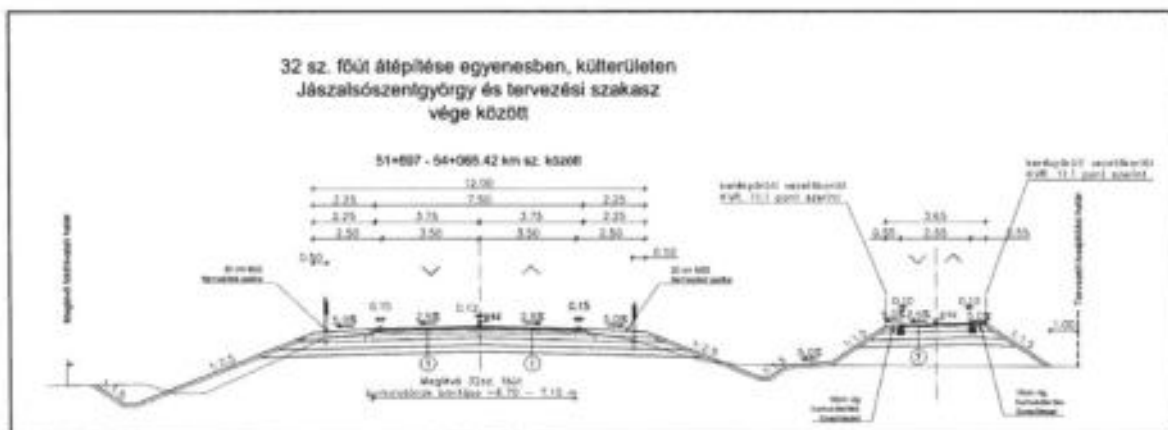
Viköti Kft V241 munkaszámú terve keresztmetszvények
