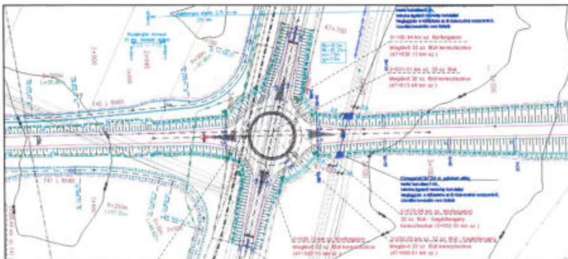
Viköti Kft V241 munkaszámú terve útépítési helyszínrajz
